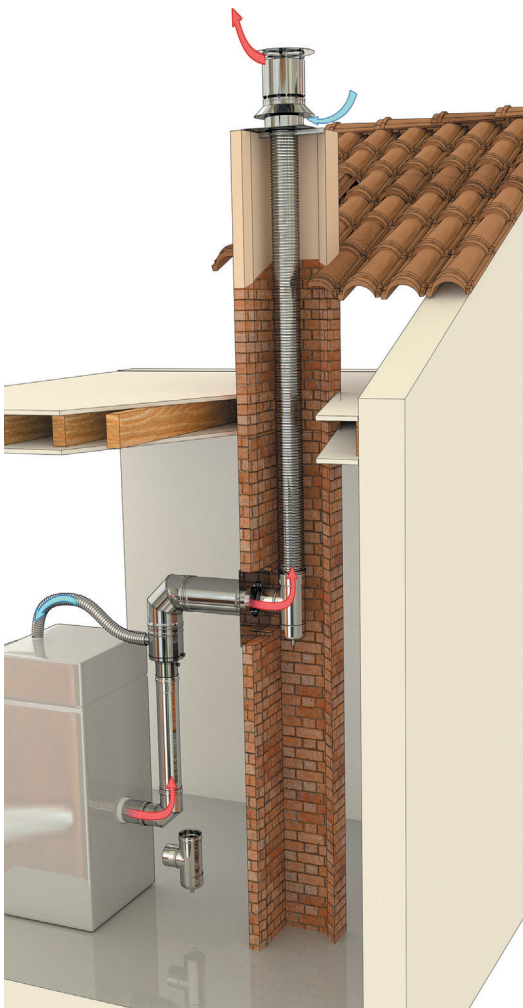
Exemple de configuration Rénovation de conduit existant - Zone 2
