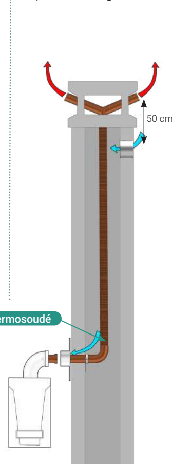
> Terminal en T pour montage C5
