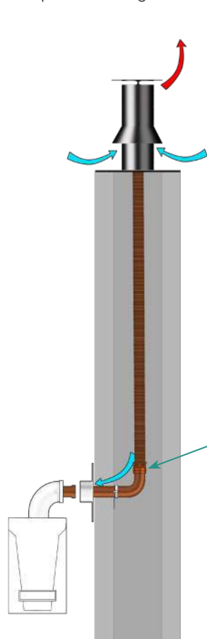
> Terminal de cheminée pour montage C9
