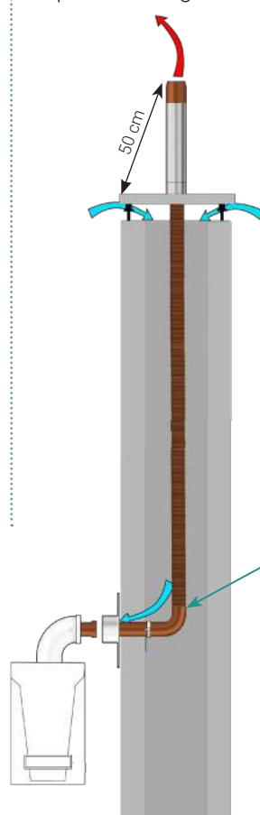
> Terminal de réhausse pour montage C5
