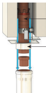
> Solution plafond exemple avec raccord
