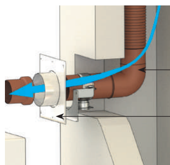
> Solution murale exemple avec coude
